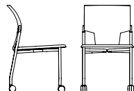
KE / KR / KP 21 BW 16" SW 16" BH 15" SH 19" SD 16.5"
