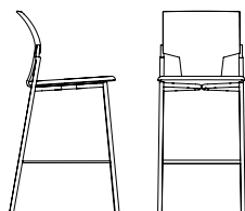
KE / KR / KP 25 BW 16" SW 16" BH 15" SH 30" SD 16.5"
