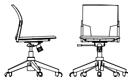
KE / KR / KP 40 BW 16" SW 16" BH 15" SH 17.5-22" SD 16.5"
