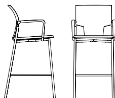
KE / KR / KP 35 BW 16" SW 16" BH 15" SH 30" SD 16.5"
