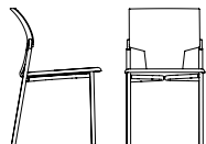
KE / KR / KP 20 BW 16" SW 16" BH 15" SH 19" SD 16.5"
