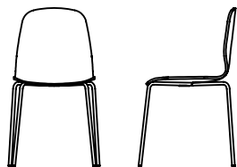
KO22 BW 16" SW 17" BH 15" SH 18" SD 18"
