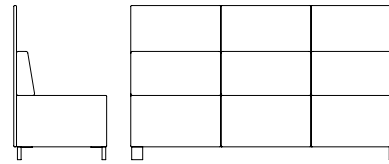
BL43P H 42" D 25" W 72"
