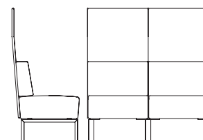
PO52P H 51" W 27" L 48"
